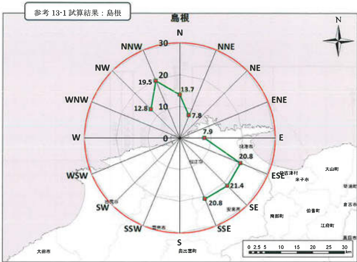
福島第一原子力発電所（1～3号機）の放射性物質質量と同じと仮定した計算
