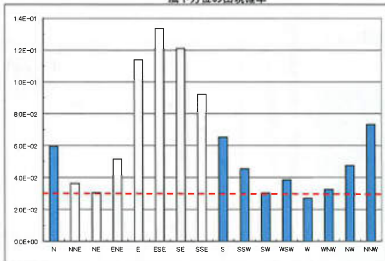
風下方位の出現確率
