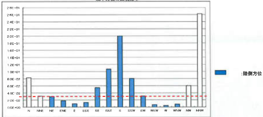
風下方位の出現確率
