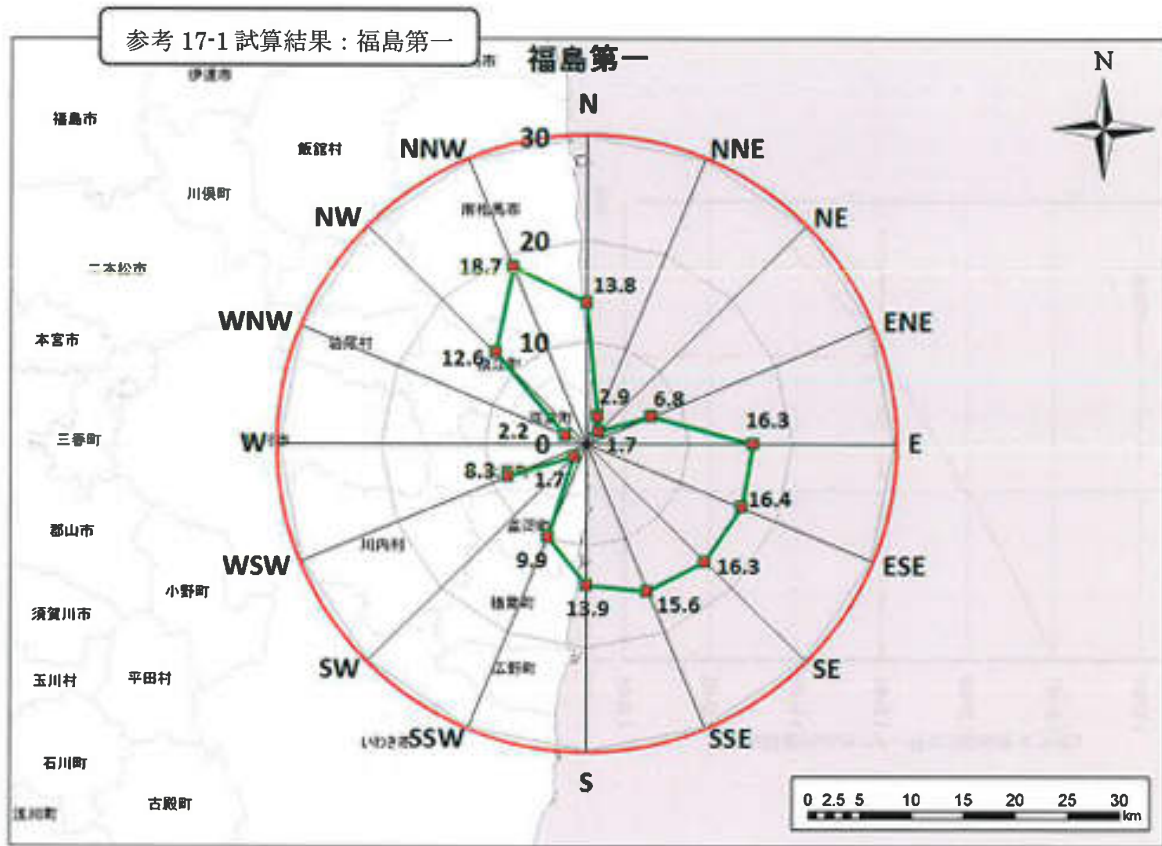
福島第一原子力発電所（1～3号機）の放射性物質量の拡散距離等を計算
