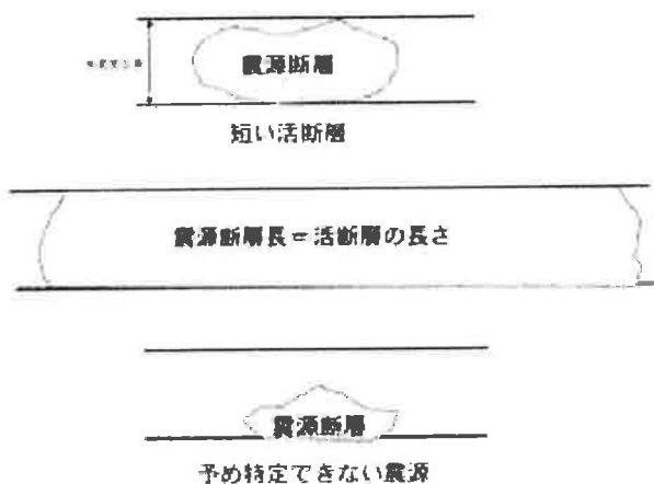
図1. 震源断層と活断層との関係[1]
