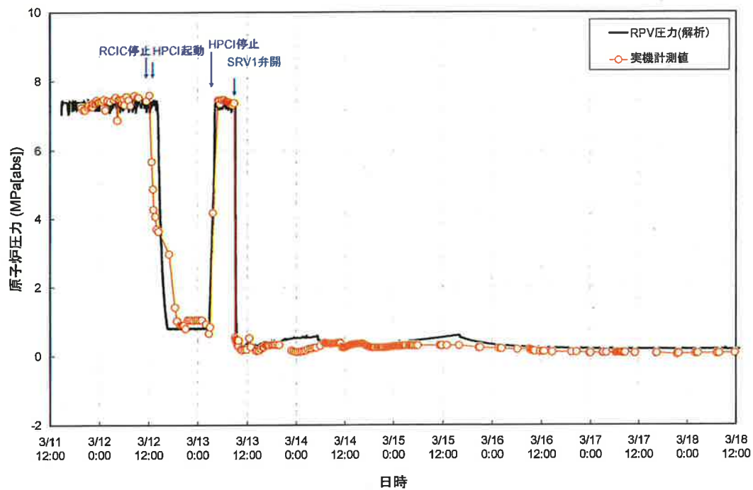
図 3. 3. 1. 10 3号機 原子炉圧力変化【その1】(蒸気漏えい)
