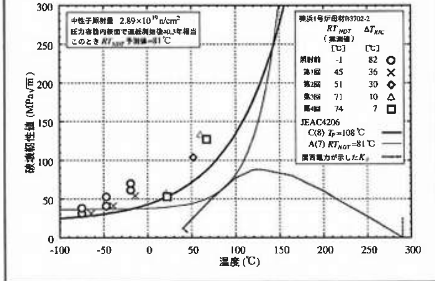
図3: PTS評価(母材B3702-2)
