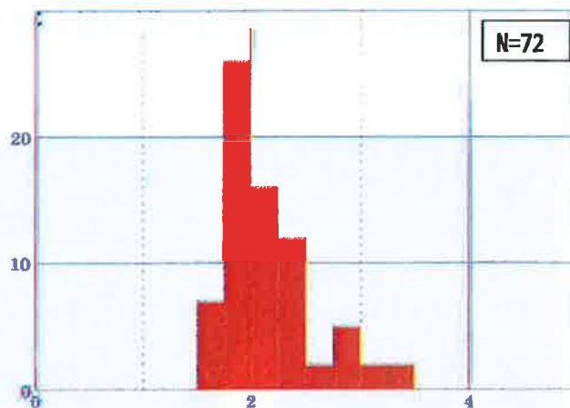
図 2.4.4 アスペリティの平均変位
